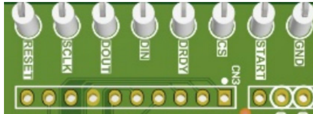
Figure 1-4 NSAD124xEVM数字接口示意图
