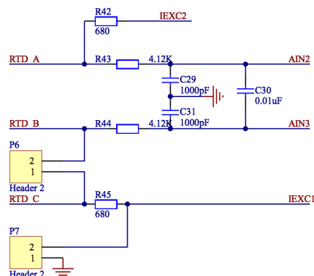
Figure 3-2 NSAD124x EVM 上的 RTD 输入结构
