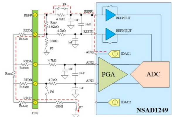
Figure 3-9 高侧基准的四线制RTD测量拓扑
